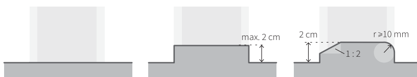
Przekrój przez próg: brak progu (rozwiązanie zalecane), próg do 2 cm, próg 2-centymetrowy z zaokrągleniem krawędzi min. 10 mm z jednej strony i fazowaniem min. 1:2 z drugiej.
